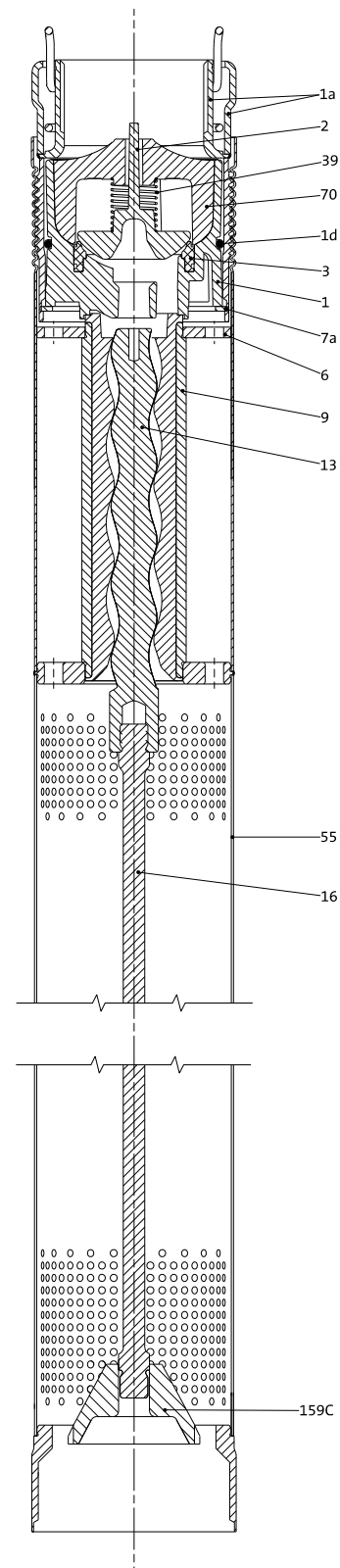
Fig. 29 Example: SQF 1.2-2
