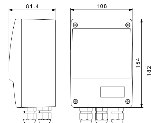
Fig. 22 Dimensions, CIU 273
